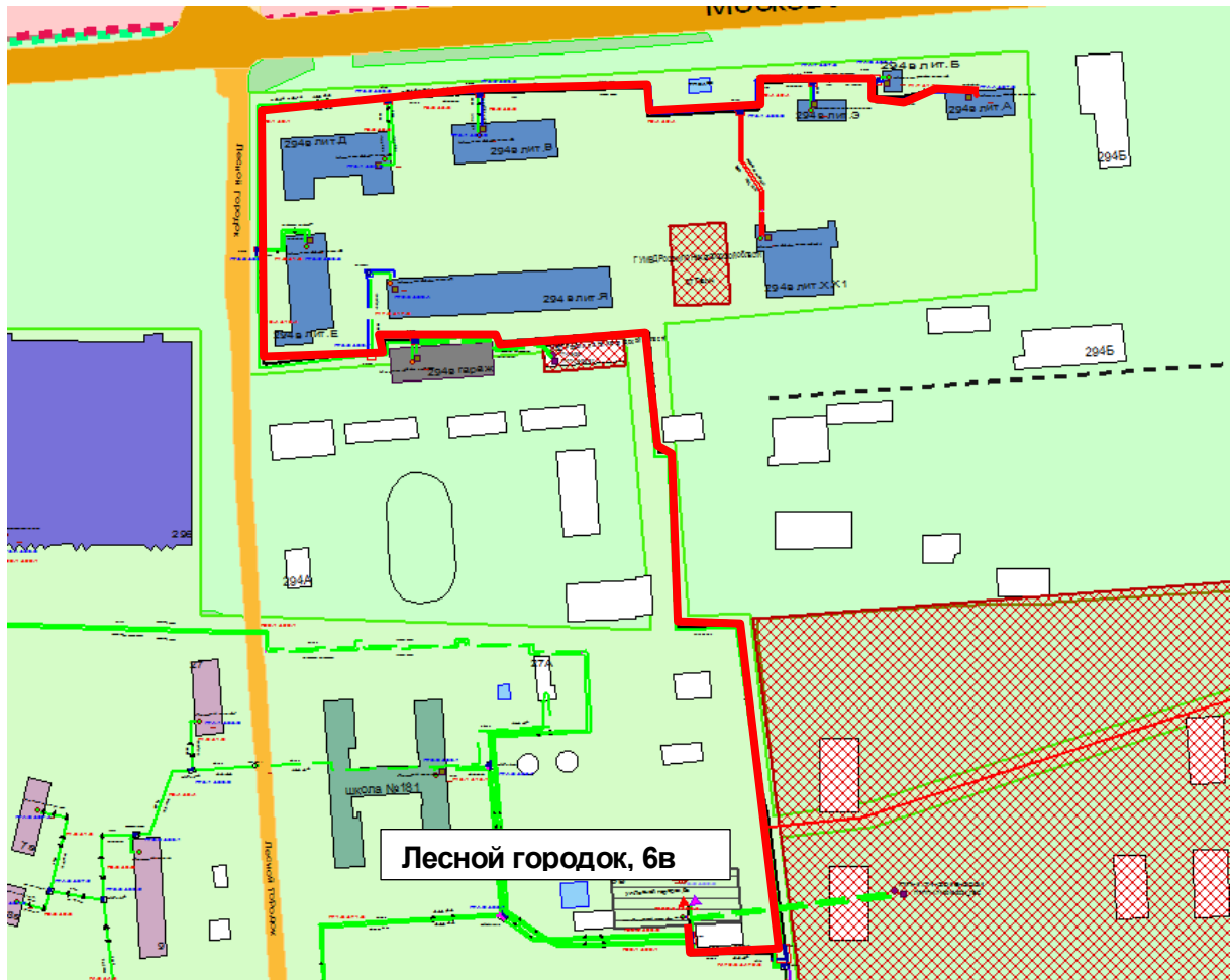
Рисунок 1.19 – Результат гидравлического расчета - расчетный путь теплоносителя от Лесной городок 6в до ПТ-Моск.ш,294в лит.А
